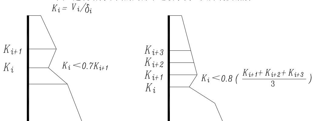
图4 沿竖向的侧向刚度不规则（有软弱层）
