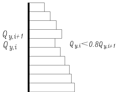
图 6 竖向抗侧力结构屈服抗剪强度非均匀化（有薄弱层）
