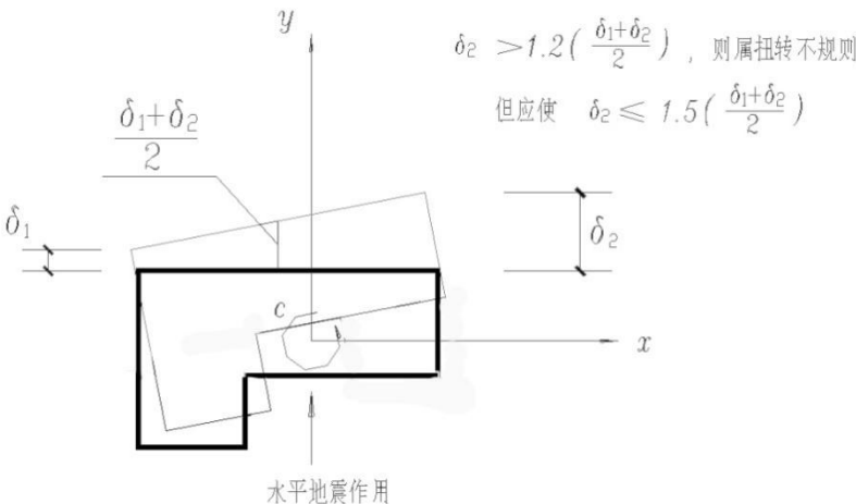
图1 建筑结构平面的扭转不规则示例
