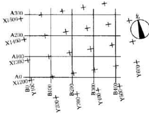
图 2.4.1 坐标网格
