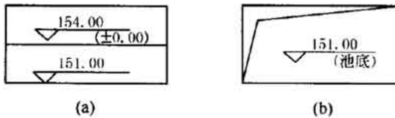
图 2.5.2 标高注法
